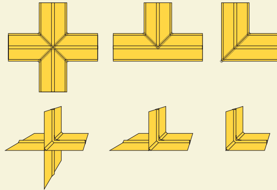
Standardformteile
